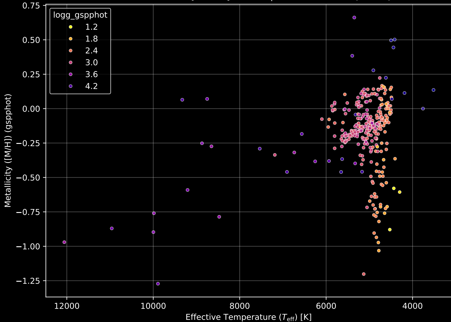
APOGEE DR17 Field: [240+00] Stellar Population Parameters (n= 331)
